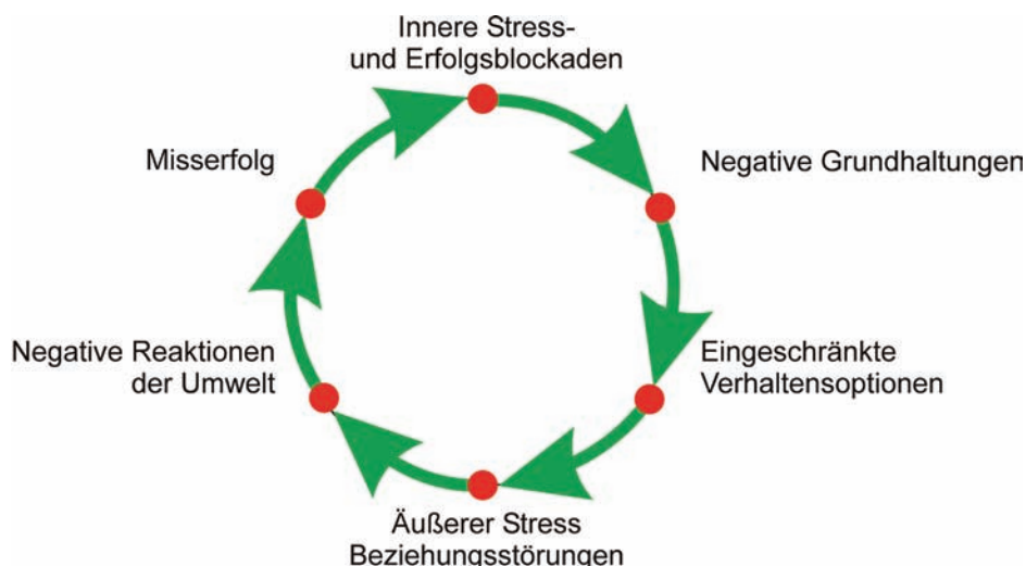
Abbildung 2: Stress-Spirale
